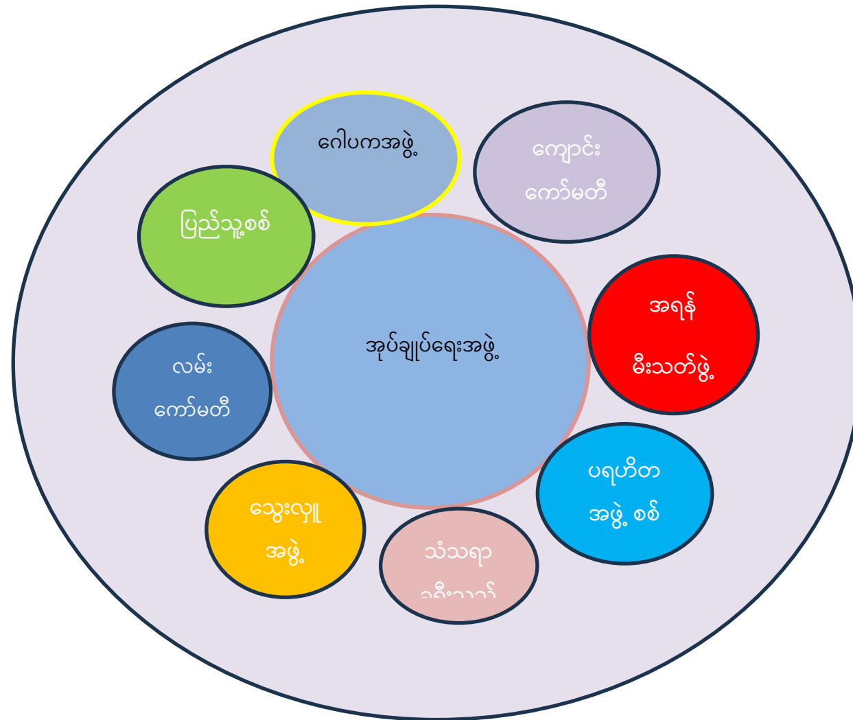
Venn Diagram
